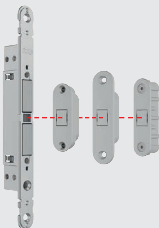
Alineamiento Touch con soportes Minimal-Touch , Easy-Touch y Alu-Touch .
