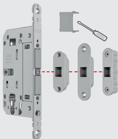
Alineamiento de Touch & Close con soportes Minimal-Touch , Easy-Touch y Alu-Touch . Es necesario quitar la tapa frontal del soporte para permitir el alojamiento del pasador en posición de cierre.
